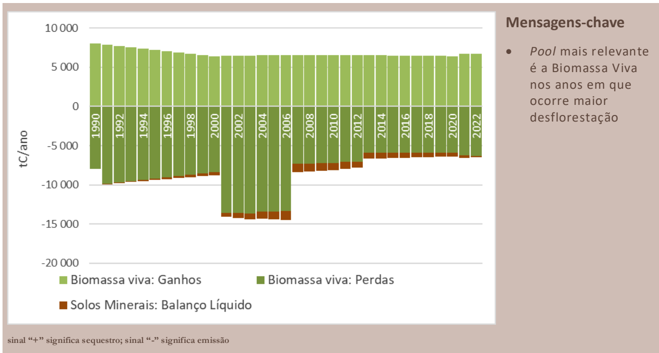
Figura 49: Emissões / Sequestro da Categoria 4B Agricultura: por pool
