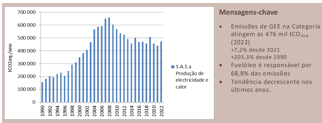
Figura 16: Emissões da Queima de Combustíveis na Produção de Electricidade e Calor
