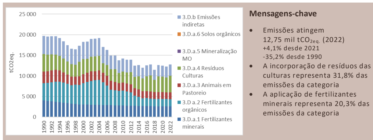
Figura 34: Emissões Solos Agrícolas
