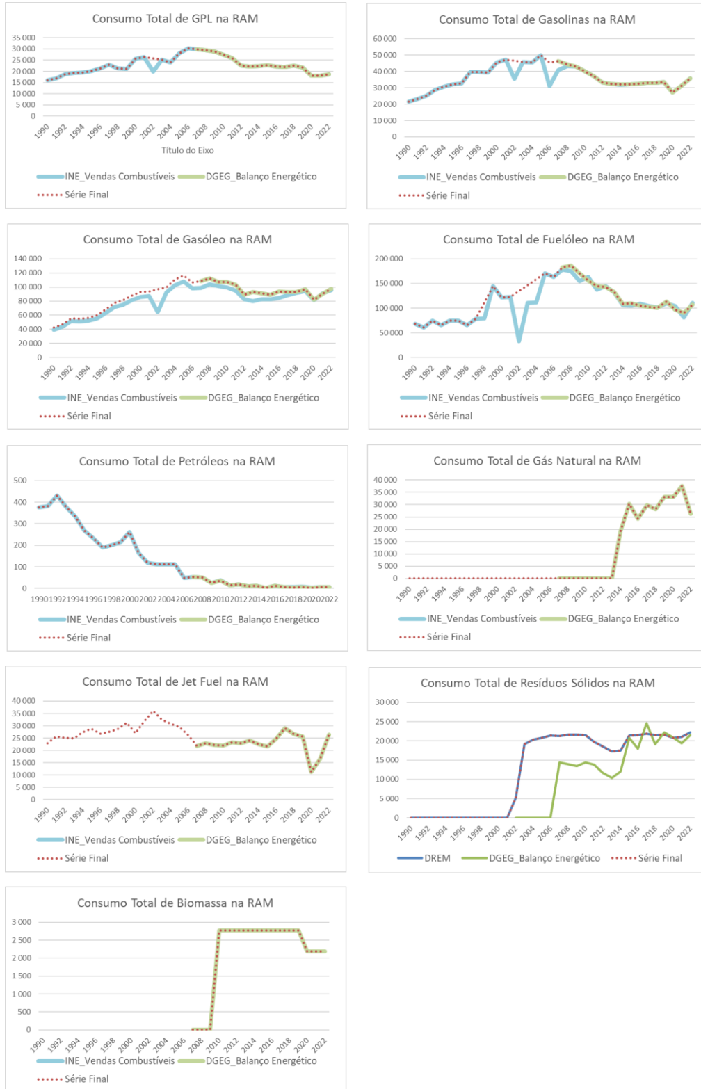
Figura 10: Consumos Totais por Combustível (tep/ano) – séries de dados originais e final
