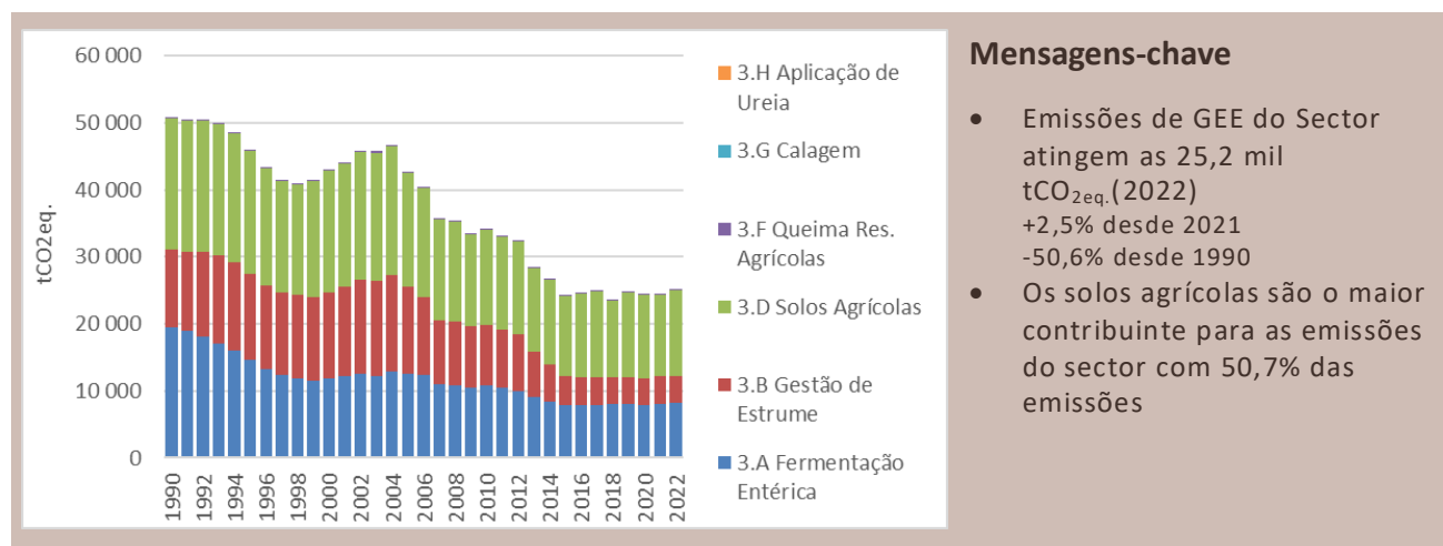
Figura 24: Evolução das Emissões do Sector Agricultura
